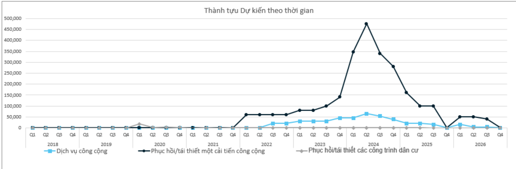
Hình 49: Thành tựu Dự kiến theo thời gian
